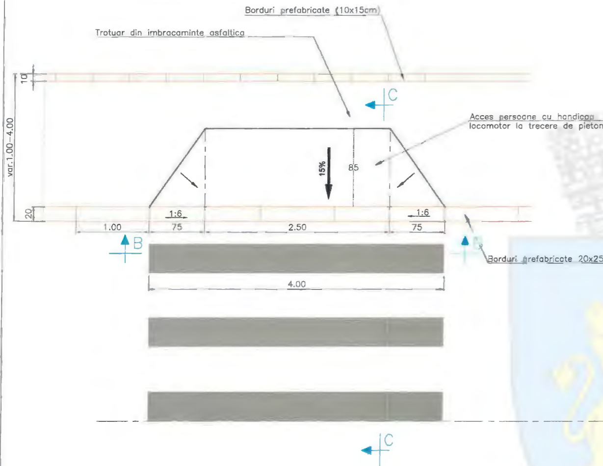
VEDERE A-A Sc: 1:50
