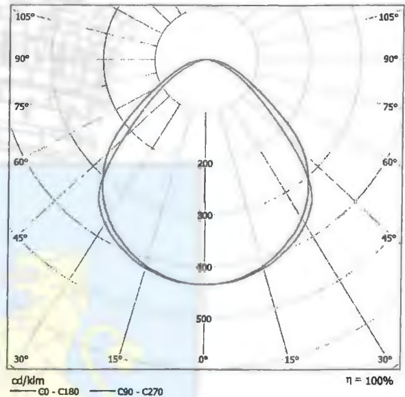
Distribuția luminoasă 1:
