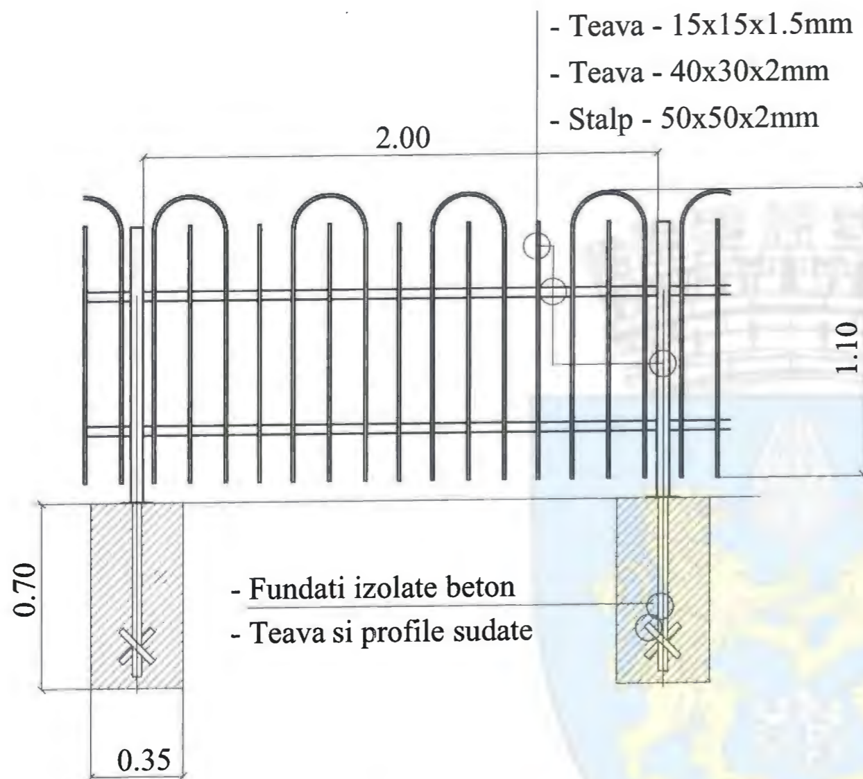
VEDERE 1/20
