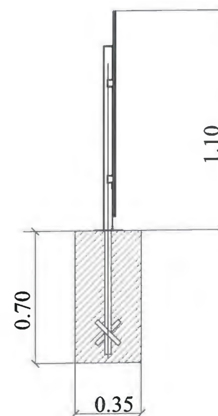
SECTIUNE 1/20
